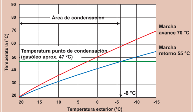
Ejemplo: Radiadores (dimensionado 70/55 °C)
