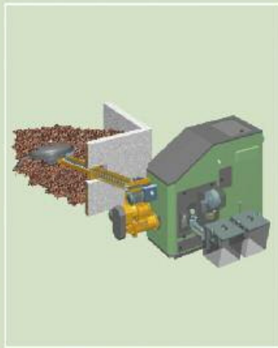
Alimentación totalmente automática de una cadena de recortes de leña
