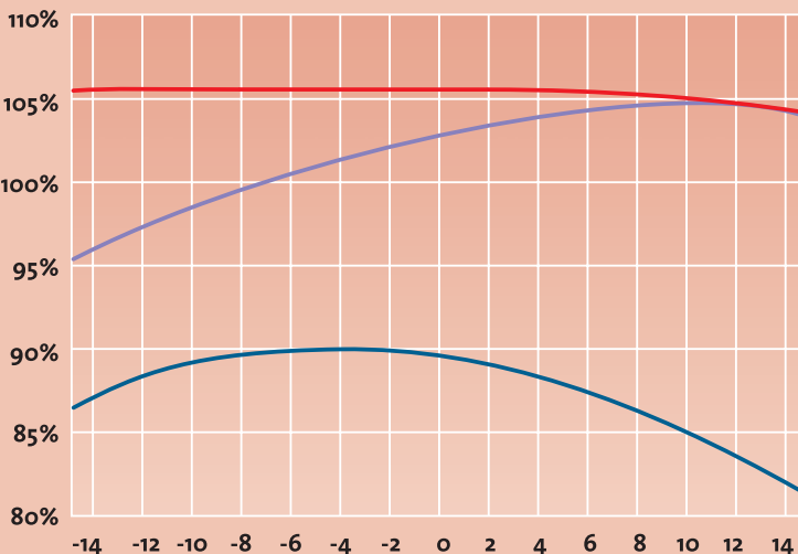
Comparación de efectividad entre caldera de condensación y caldera de baja temperatura
