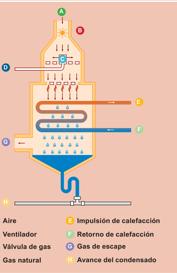
Esquema de un aparato de condensación
