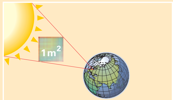
1.367 W/m 2 potencia de radiación al penetrar en la atmósfera terrestre
