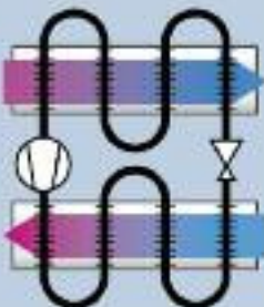
Bomba de calor del aire de salida
