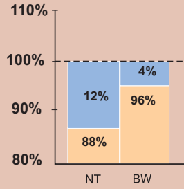
Parámetro valor calorífico H_i Parámetro valor calorífico bruto H_s
