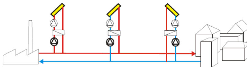
Ilustración 44. Esquemas generales de conexión a red urbana
