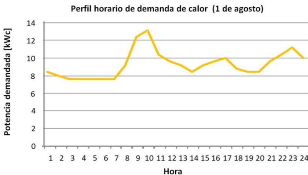
Ilustración 57. Perfil horario de demanda de calor en Ecoenergías (1 de agosto)
