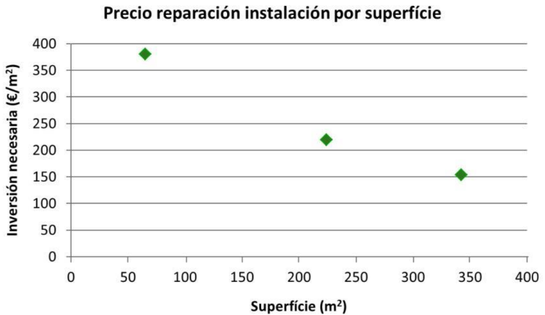
Ilustración 86. Precio reparación instalación por superficie. Fuente: AIGUASOL
