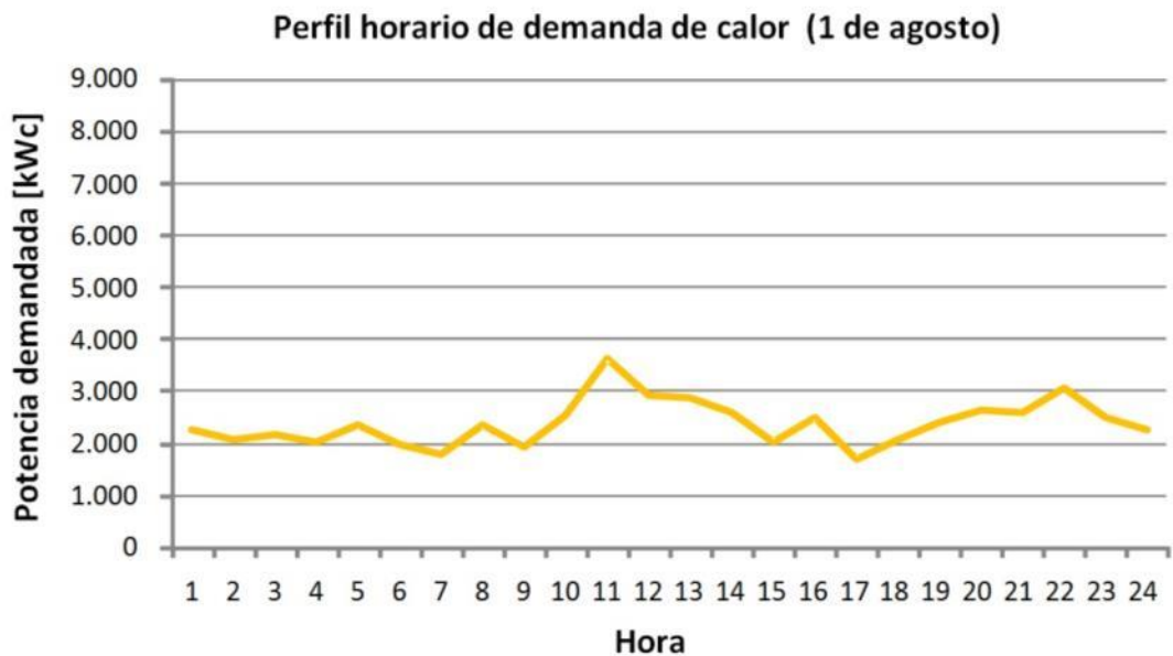
Ilustración 55. Perfil horario de demanda de calor en Districlima (1 de agosto)
