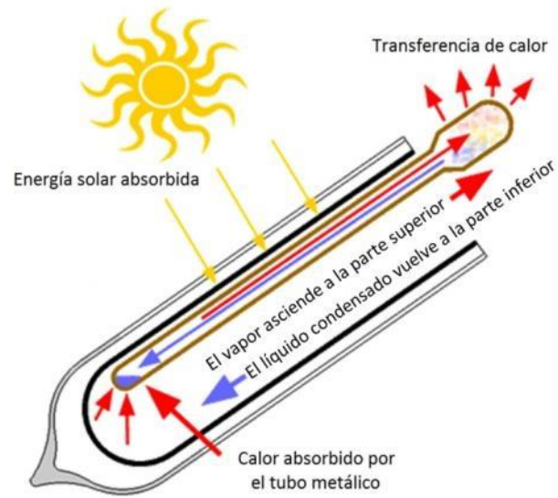
Ilustración 24. Colector de tubo de vacío Heat pipe. Fuente: APRICUS-SOLAR
