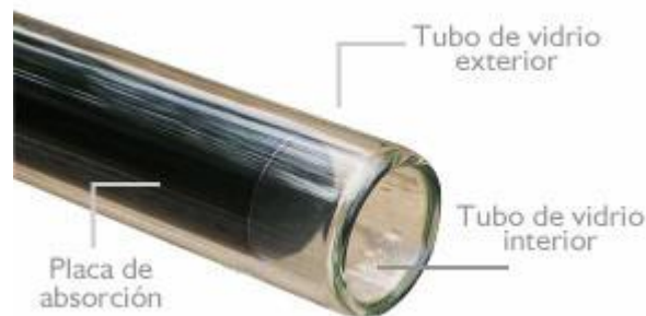
Ilustración 22. Tipos colectores de flujo directo: tubos de vacío vidrio-vidrio (glass-glass pipes, en inglés). Fuente: APRICUS-SOLAR
