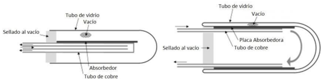
Ilustración 21. Ejemplos de captador de tubo de vacío con flujo directo vidrio-metal: concéntrico (izquierda) y tubos separados (derecha). Fuente: Fraunhofer ISE
