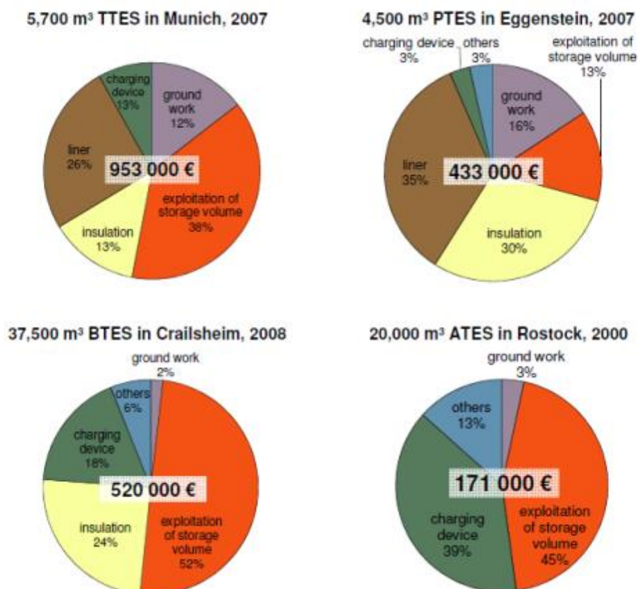
Ilustración 42. Ejemplos de costes para cada concepto, sin IVA ni ingeniería (Fuente: IEE SDH Guidelines)
