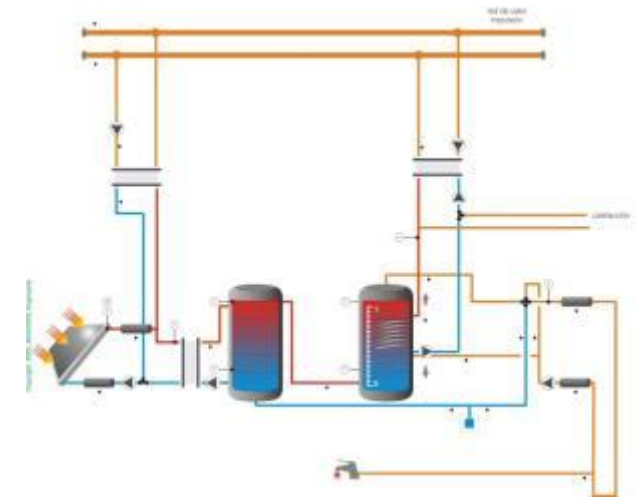
Ilustración 91. Esquema de principio conexión 1 (SCH1)
