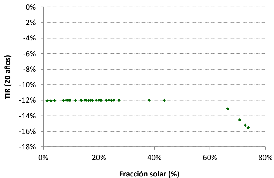
Ilustración 72. TIR en función de la demanda anual para el SST de con LFC instalado en Disticlima
