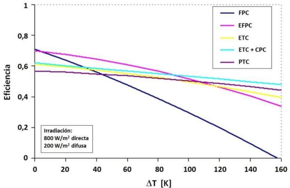
Ilustración 31. Rendimiento de distintos captadores en función de la diferencia de temperatura con el ambiente
