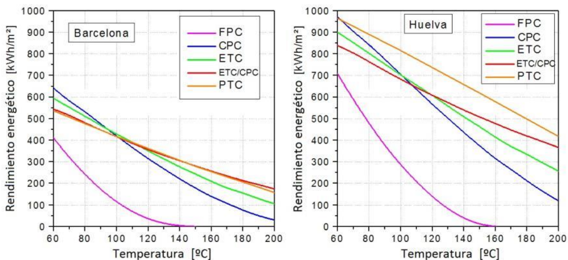
Ilustración 32. Rendimientos típicos de captadores de energía bruta como función de la temperatura de salida del captador, calculados para instalaciones en Barcelona y Huelva, España
