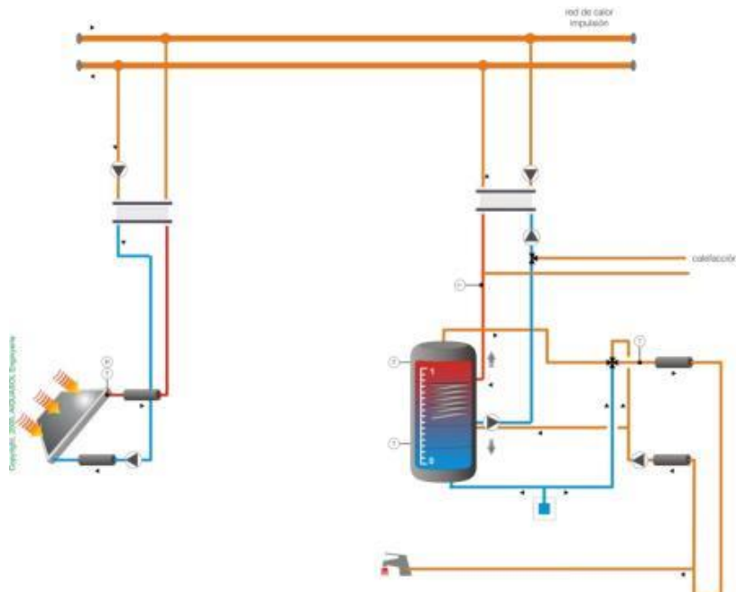
Ilustración 85. Esquema de principio conexión 3 (SCH3)
