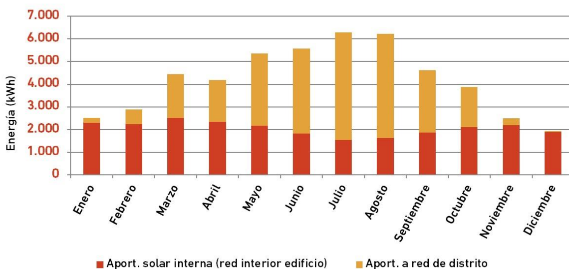
Ilustración 81. Aportación calor a la red e interior SCH1 TIP1
