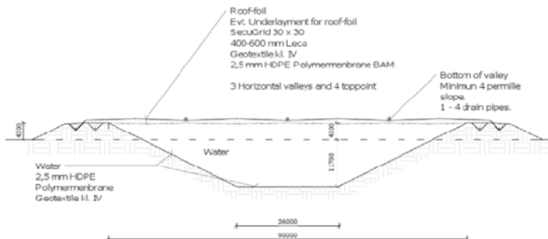
Ilustración 37. Sección transversal de los 75.000 m 3 PTES en Marstal. (Fuente: PlanEnergi)
