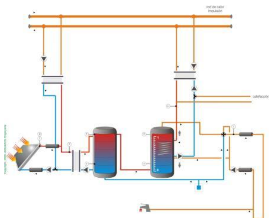
Ilustración 79. Esquema de principio conexión 1 (SCH1)
