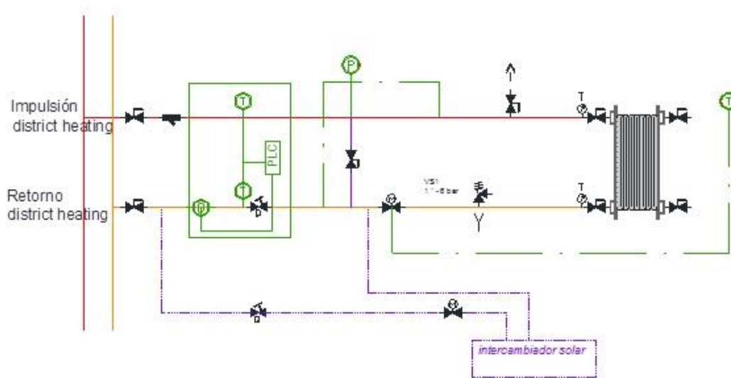
Ilustración 88. Esquema de detalle conexión 2 (SCH2)
