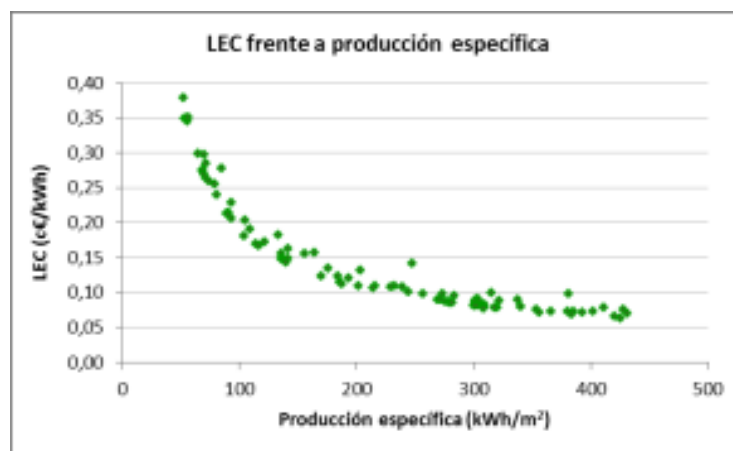
Ilustración 5. Evolución del LEC [c€/kWh] en función de la producción específica [kWh/m²]
