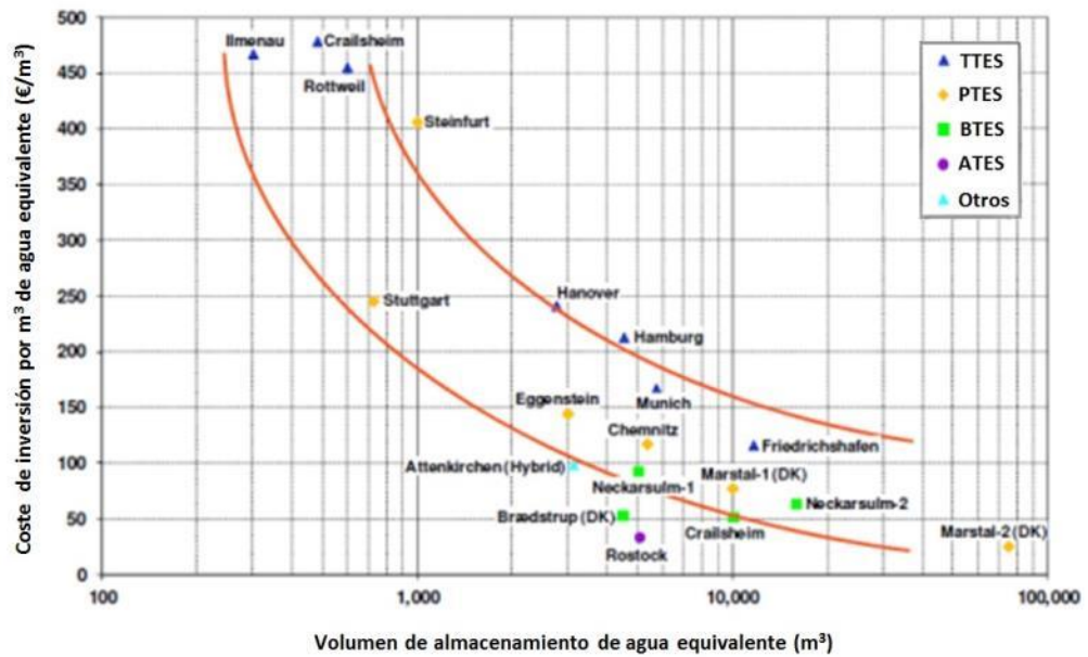
Ilustración 43. Costes específicos de proyectos de demostración sin IVA. Referencias sin código son Alemania. (Fuente: IEE SDH Guidelines)
