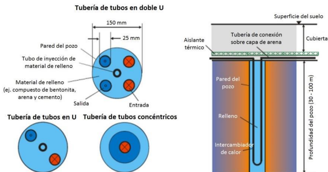
Ilustración 39. Tipos más comunes y la sección vertical de sondas geotérmicas. (Fuente: ITW, Universidad de Stuttgart)
