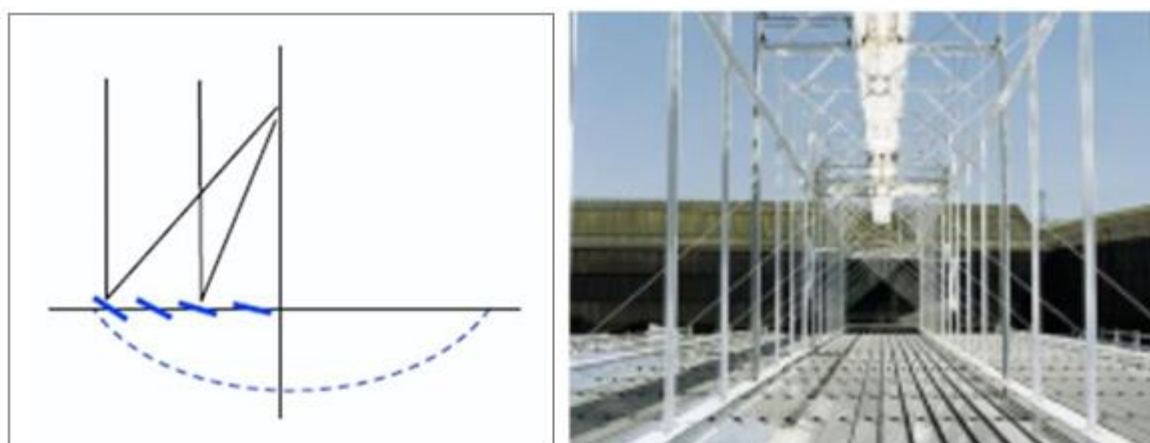
Ilustración 29. Trazado de rayos y vista general de un Captador Lineal de Fresnel
