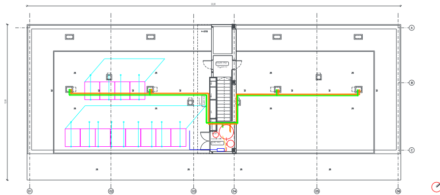
Ilustración 78. Planta cubierta edificio existente
