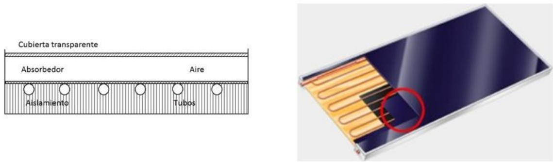
Ilustración 18. Sección lateral de un colector solar plano (izquierda). Detalle de un colector solar plano (derecha). Fuente: VIESSMANN
