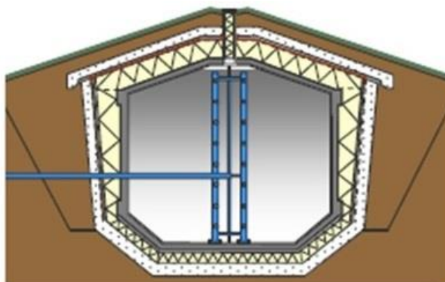
Ilustración 35. Tanque de almacenamiento de energía térmica (TTES en inglés)
