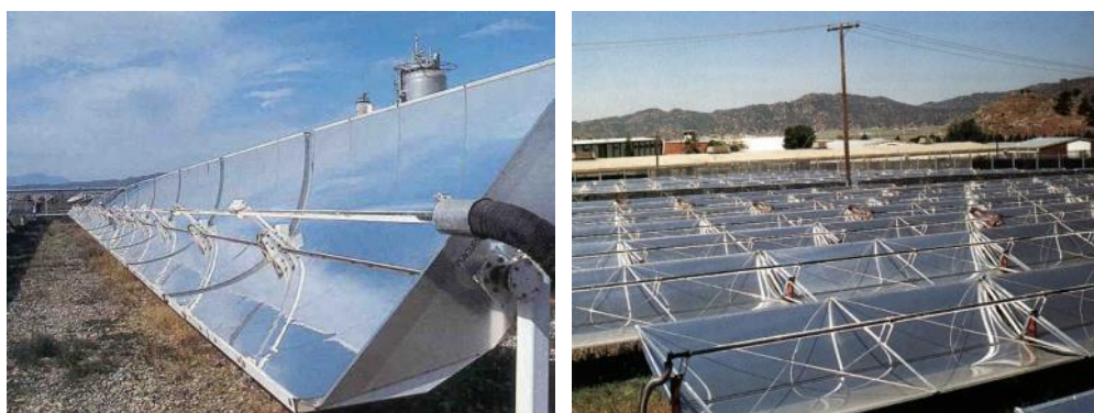
Ilustración 28. Colectores cilindro-parabólicos con un eje de orientación este-oeste (izquierda). Aplicación de colectores cilindro-parabólicos en un proceso industrial (derecha)
