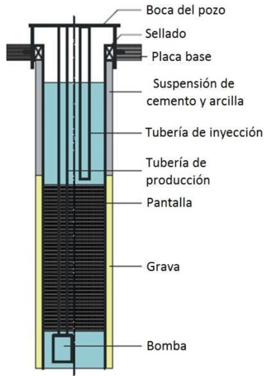
Ilustración 41. Diseño de un pozo para carga y descarga. (Fuente: Geothermie Neubrandenburg GmbH)
