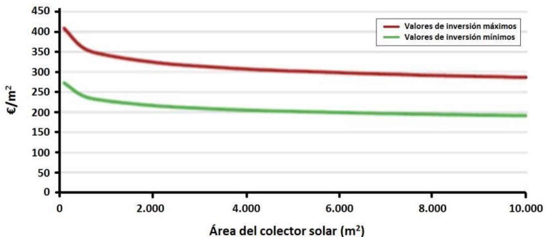
Ilustración 50. Coste de circuito primario instalado considerado en el estudio
