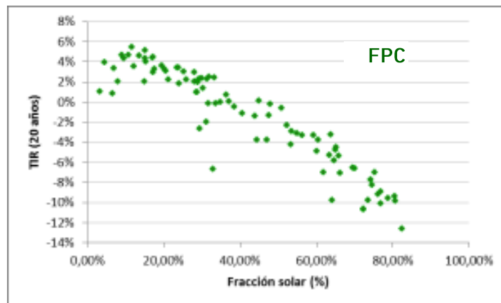
Ilustración 1. Tasas Internas de Retorno en función de la fracción solar para una instalación de FPC
