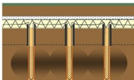
Almacenamiento de energía térmica en sondeos
