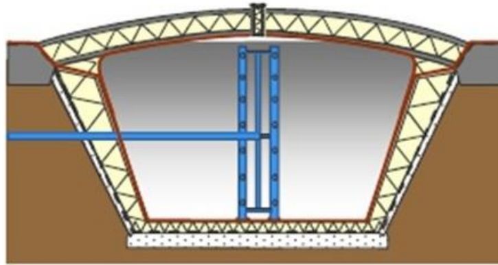
Ilustración 36. Almacenamiento de energía térmica en pozo (PTES en inglés)
