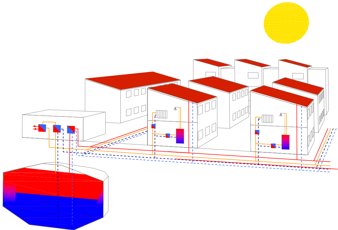
Ilustración 48. Esquema hidráulico de una red distribuida, con doble red. Fuente : Solites
