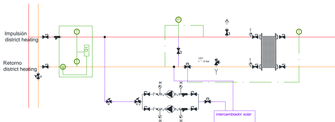
Ilustración 89. Esquema de detalle conexión 3 (SCH3)
