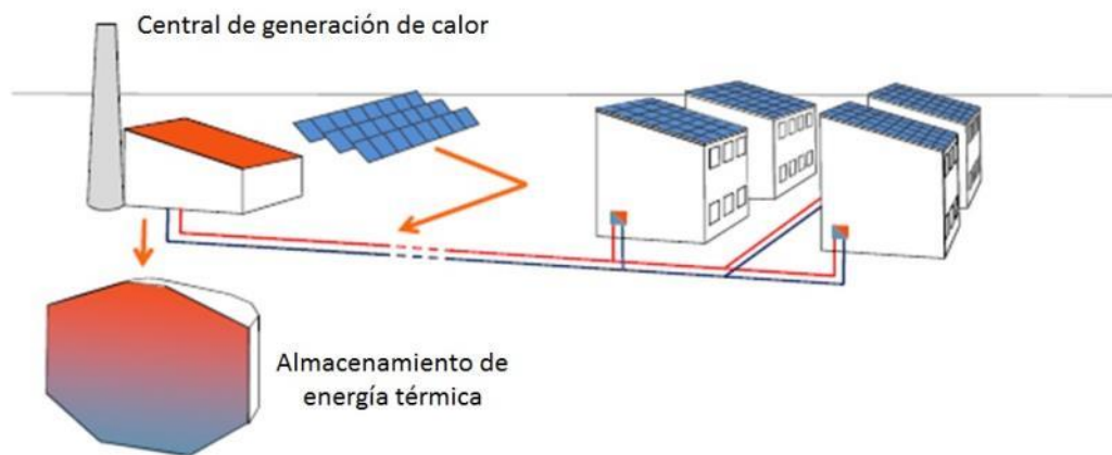
Ilustración 33. Acumulación estacional en red de distrito (Fuente: Solites)
