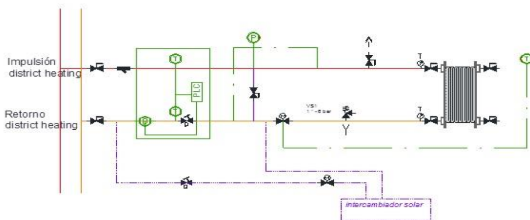
Ilustración 84. Esquema de principio conexión 2 alternativo (SCH2)
