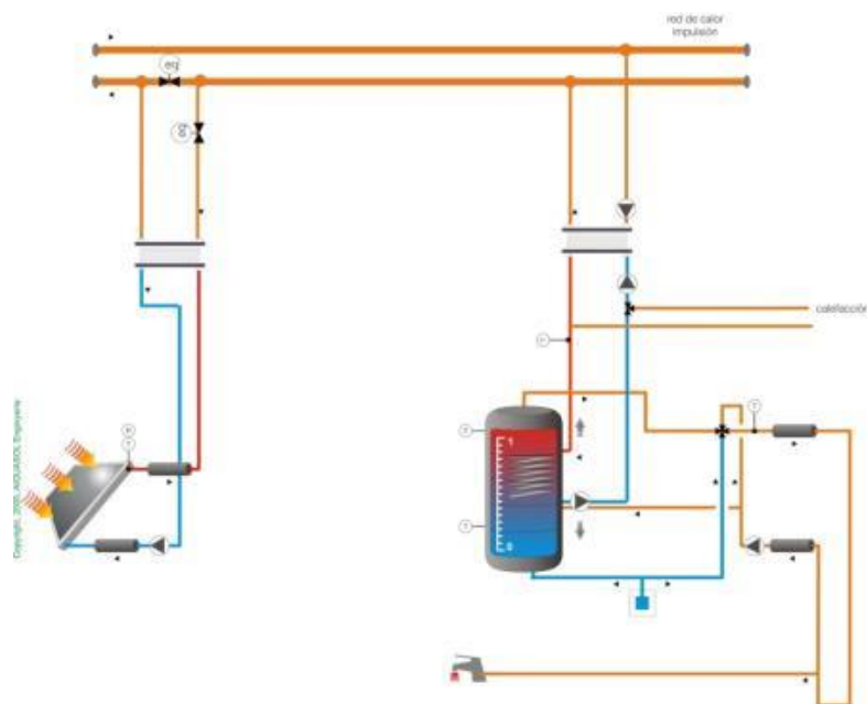
Ilustración 83. Esquema de principio conexión 2 (SCH2)
