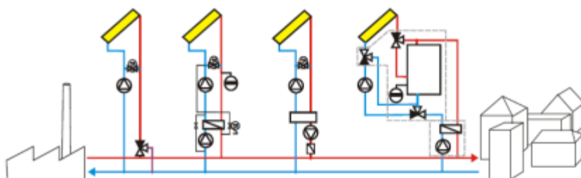
Ilustración 45. Esquemas puntuales de funcionamiento dentro del campo solar
