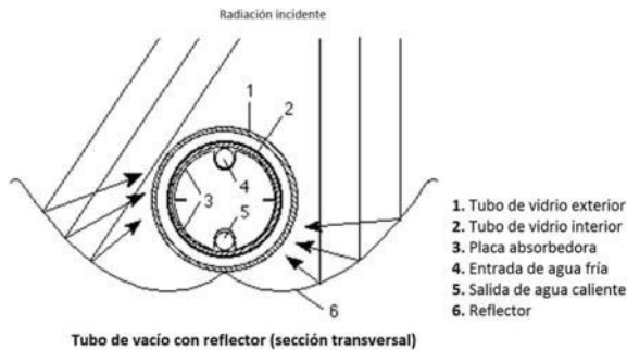
Ilustración 23. Colector tipo Sydney con reflector CPCP (izquierda). Fuente: MICROTHERM Energietechnik GmbH. Colector de tubos concéntricos con reflector en el interior del tubo (derecha). Fuente: SCHOTT
