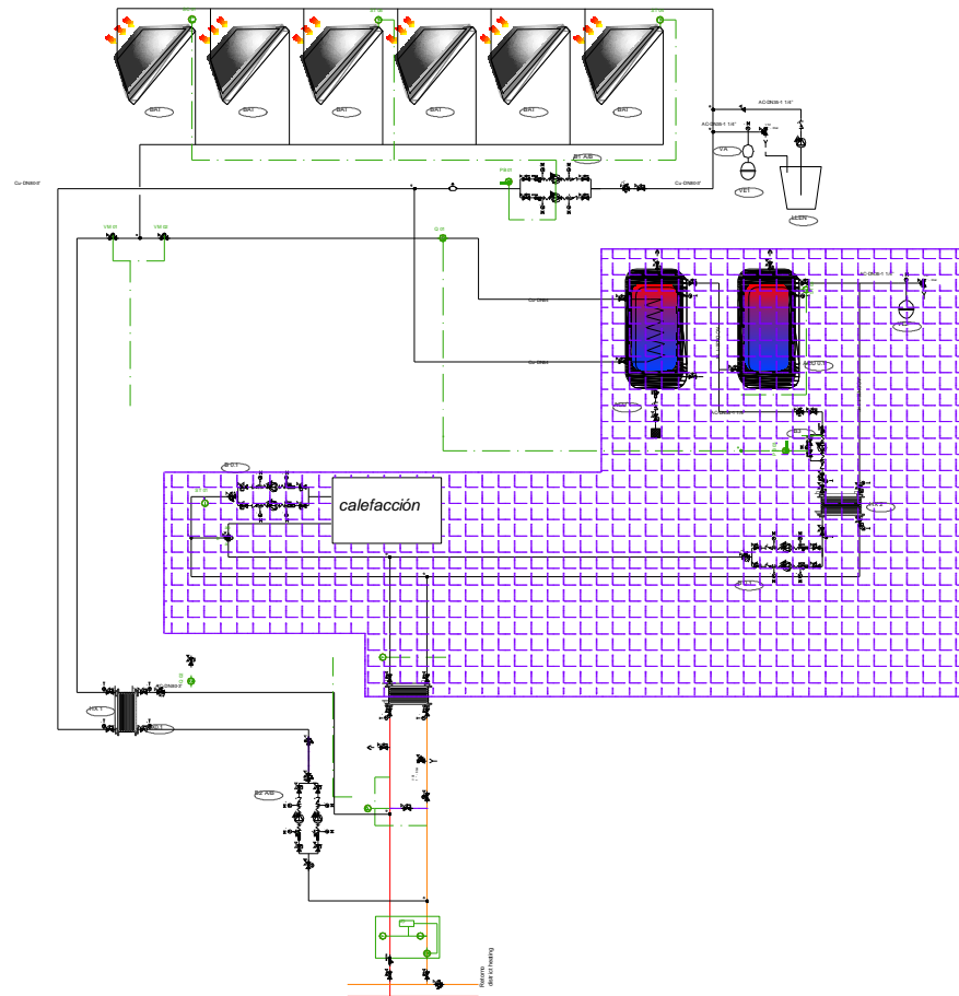
Ilustración 87. Esquema de detalle conexión 1 (SCH1) con gestión solar red de distrito
