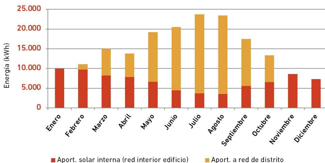
Ilustración 82. Aportación calor a la red e interior SCH1 TIP3
