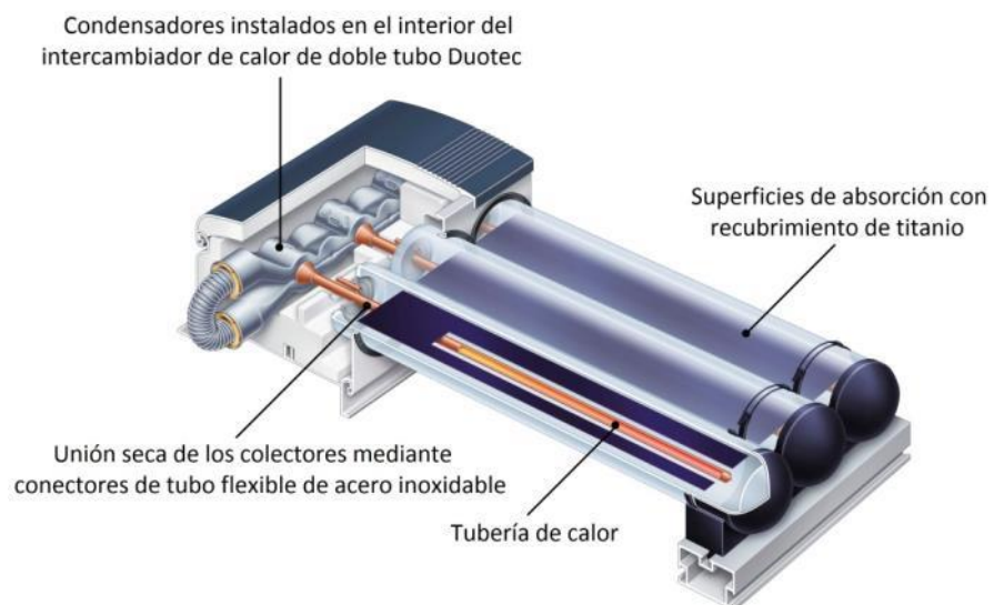
Ilustración 25. Detalle de la conexión entre el heat pipe y el circuito de agua. Fuente: VISSMANN
