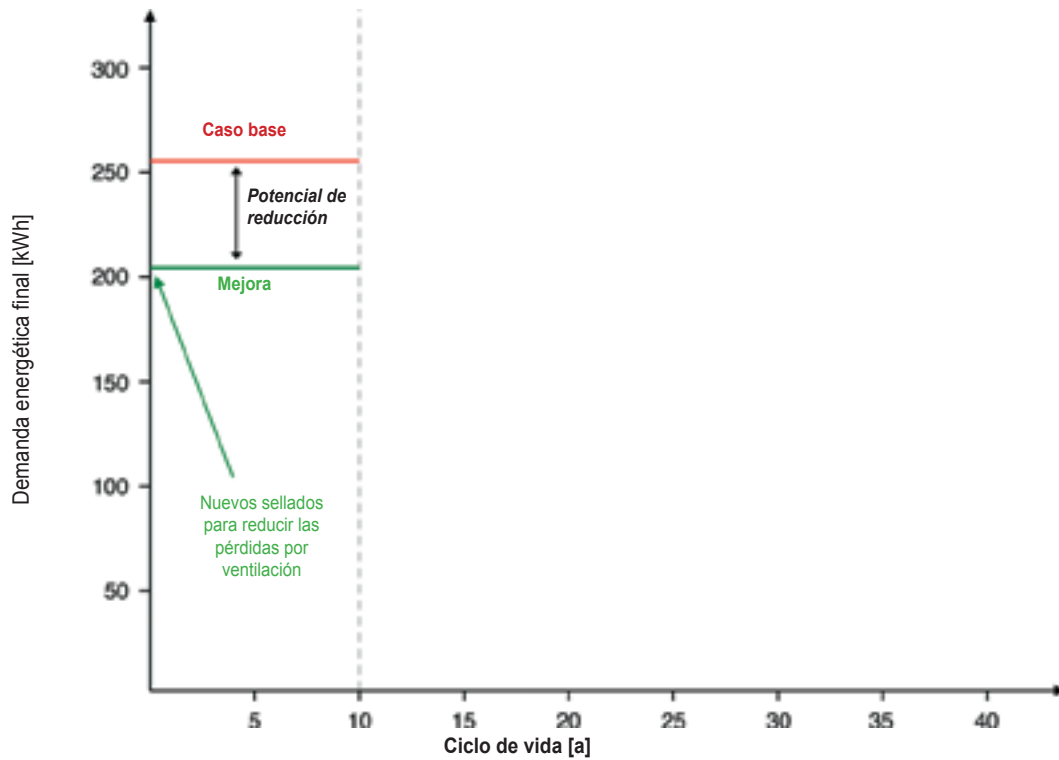
Figura 7.3 Demanda de energía final del caso base y la mejora «nuevo sellado para reducir las pérdidas por ventilación»
