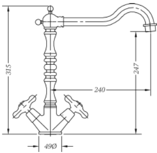
Ref.: 68595 09 43 66 Monobloc de fregadera bronce Bronze sink mixer
