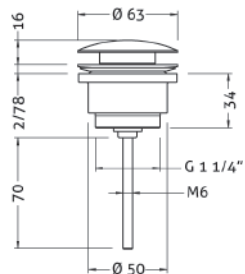
Ref.: 100211 45 Válvula click "Luxe" 1 1/4" 1 1/4" "Luxe" click valve
