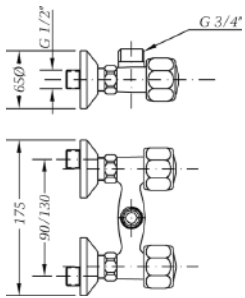
Ref.: 568195 45 Cuerpo grupo mural 11 cm Wall body mixer 11 cm
