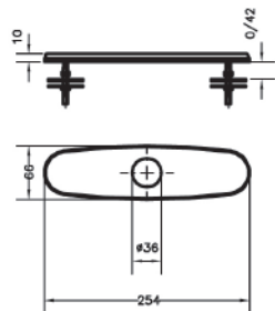
Ref.: P200 Placa adaptadora 8" 8" adaptor plate
