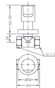
Ref.: 68170 07 45 66 Llave de paso 1/2" Stopcock 1/2"
