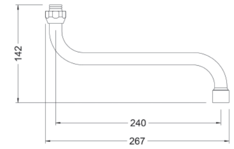
Ref.: 68904 45 Caño bajo tubo 24 cm Low tube spout 24 cm
