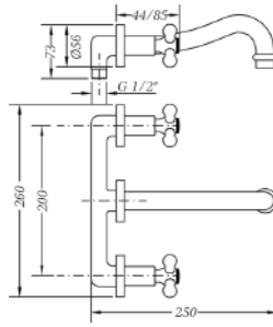
Ref.: 68131 09 45 66 Grupo de lavabo empotrado Built-in wash-basin mixer
