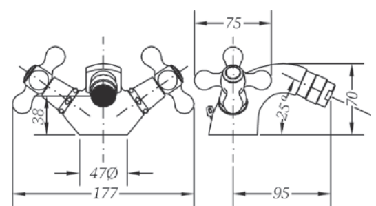
Ref.: 68515 09 45 66 Monobloc de bidé Bidet mixer
