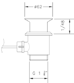
Ref.: 100200 45 Válvula automática plástico 1 1/4" 1 1/4" plastic automatic valve
