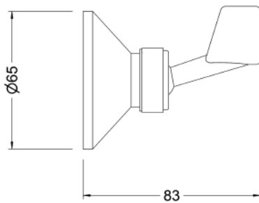
Ref.: 1647 45 Soporte ducha Clásico Classic shower holder
