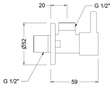
Ref.: 3104 05 Válvula de escuadra redonda 1/2" Round angle valve 1/2"
