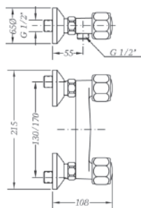
Ref.: 68110 11 45 66 Mezclador de ducha con kit Shower mixer with kit
