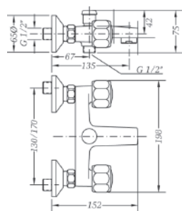
Ref.: 68100 11 45 66 Mezclador de baño con kit Bath mixer with kit
