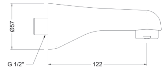
Ref.: 1667 45 Caño mural baño fundido Casted wall bath spout
