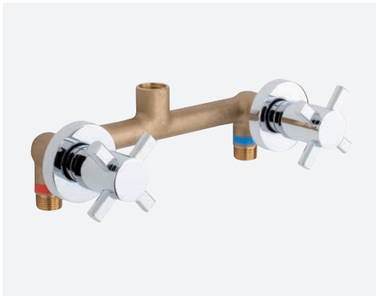
Ref.: 68115 08 45 66 Grupo ducha empotrado 8" Built-in 8" shower mixer
