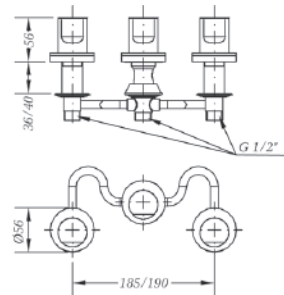
Ref.: 68142 07 45 66 Batería de bidé con transmisión Widespread bidet mixer with transmission
