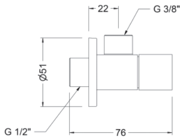
Ref.: 3106 05 Válvula de escuadra cuadrada 1/2" Square angle valve 1/2"
