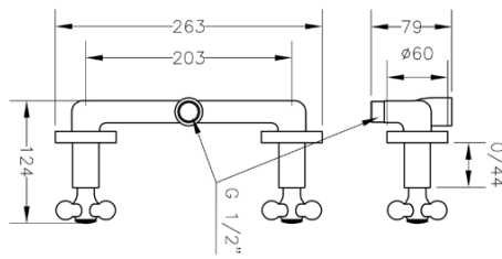
Ref.: 68535 09 45 66 Grupo ducha empotrado 8" Built-in 8" shower mixer
