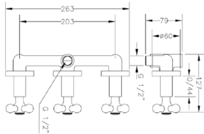
Ref.: 68527 09 45 66 Grupo baño empotrado 8" con inversor Built-in 8" bath mixer with diverter
