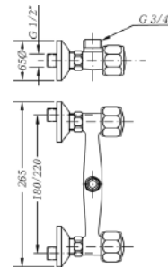
Ref.: 568104 45 Cuerpo grupo mural 20 cm Wall body mixer 20 cm
