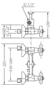
Ref.: 68531 09 45 66 Mezclador de ducha cromo con kit Chromed shower mixer with kit
