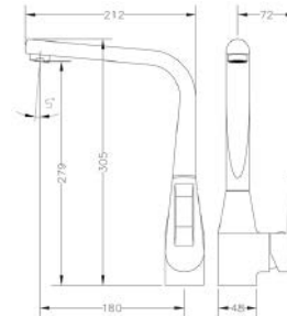
Ref.: 64201 14 45 66 Monomando de fregadera Single lever sink mixer
