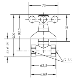
Ref.: 68590 09 45 66 Llave de paso 1/2" Stopcock 1/2"
