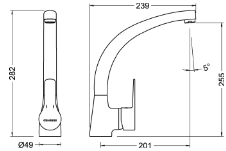
Ref.: 61203 28 45 66 Monomando de fregadera caño conformado Single-lever sink mixer tube spout
