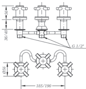
Ref.: 68142 08 45 66 Batería de bidé con transmisión Widespread bidet mixer with transmission
