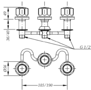
Ref.: 68142 11 45 66 Bateria de bidé con transmisión Widespread bidet mixer with transmission
