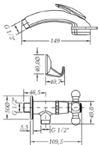
Ref.: 68001 09 45 66 Grifo de bidé con teleducha Bidet tap with shower
