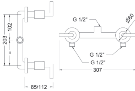
Ref.: 68115 07 45 66 Grupo ducha empotrado 8" Built-in 8" shower mixer
