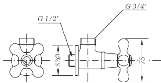
Ref.: 568575 45 Cuerpo grifo mural Wall body tap
