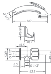
Ref.: 68001 11 45 66 Grifo de bidé con teleducha Bidet tap with shower
