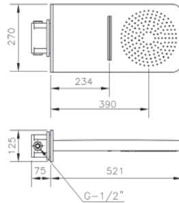
Ref.: 1643 45 Rociador doble función cascada-lluvia Shower head double function waterfall-rain
