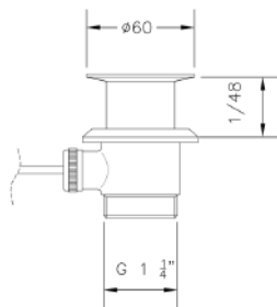
Ref.: 100203 45 Válvula automática metálica 1 1/4" 1 1/4" metallic automatic valve
