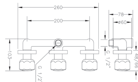
Ref.: 68116 11 45 66 Grupo baño empotrado 8" con inversor Built-in 8" bath mixer with diverter
