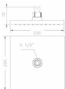
Ref.: R63112 26 Rociador cuadrado 22 cm Square shower head 22 cm
