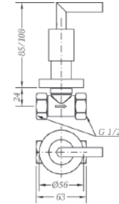
Ref.: 68170 12 45 66 Llave de paso 1/2\"/>
