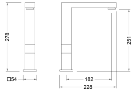
Ref.: 65208 18 60 66 Monomando de fregadera inox con cartucho progresivo Stainless steel sink mixer with progressive cartridge
