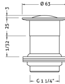
Ref.: 100207 45 Válvula click 1 1/4" 1 1/4" click valve
