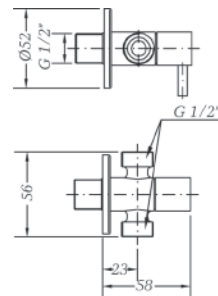
Ref.: 3108 04 Válvula de escuadra doble 1/2" - 1/2" Inox SS double angle valve 1/2" - 1/2"
