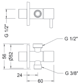
Ref.: 3107 04 Válvula de escuadra doble 1/2" - 3/8" ducha- inodoro Double angle valve 1/2" - 3/8"
