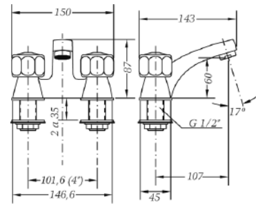
Ref.: 68122 11 45 66 Mezclador lavabo 4" Wash-basin mixer 4"
