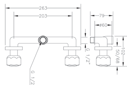
Ref.: 68115 11 45 66 Grupo ducha empotrado 8" Built-in 8" shower mixer
