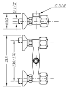
Ref.: 568193 45 Cuerpo grupo mural 15 cm Wall body mixer 15 cm
