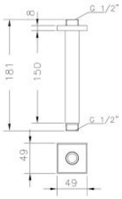
Ref.: 1672 45 Brazo a techo cuadrado 15 cm Square roof arm 15 cm
