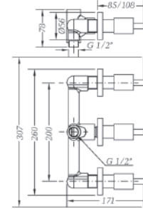
Ref.: 68116 12 45 66 Grupo ducha empotrado 8\"/>
