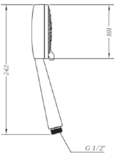
Ref.: DXK3 45 Mango de ducha K3 jets K3 jets handshower
