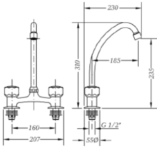
Ref.: 68194 11 45 66 Mezclador mesada 6" caño tubo 6" deck mixer with swan neck spout
