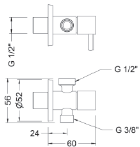
Ref.: 3107 03 Válvula de escuadra doble 1/2" - 3/8" Inox SS double angle valve 1/2" - 3/8"
