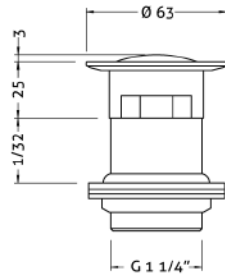
Ref.: 100206 45 Válvula click 1 1/4" con rebodadero 1 1/4" click valve with overflow
