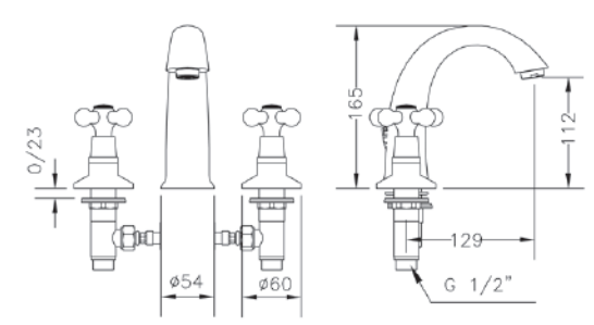
Ref.: 68120 09 45 66 Batería lavabo Widespread wash-basin mixer
