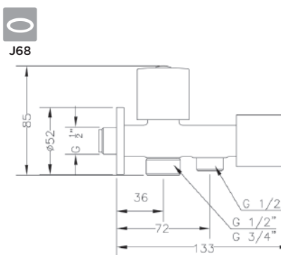
Ref.: 1023 04 Grifo doble combinable 1/2\"/>
