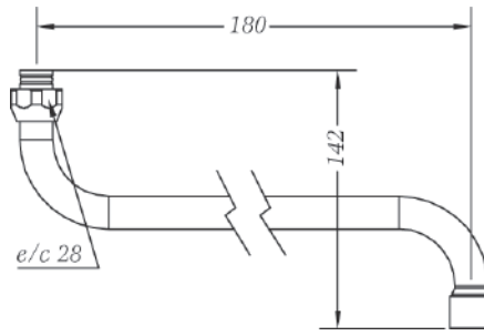
Ref.: 68910 45 Caño bajo tubo 18 cm Low tube spout 18 cm
