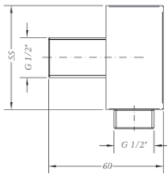
Ref.: 1679 04 Toma ducha mural cuadrada Square wall flexible connector
