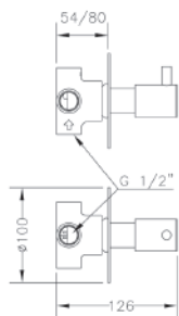
Ref.: 63114 30 45 66 Inversor cerámico 3 vías empotrado placa redonda Built-in 3 way ceramic diverter with round plate
