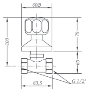
Ref.: 68170 11 45 66 Llave de paso 1/2" Stopcock 1/2"
