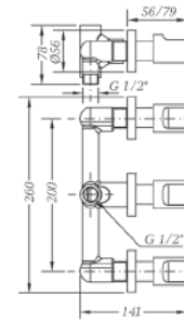
Ref.: 68116 07 45 66 Grupo baño empotrado 8" con inversor Built-in 8" bath mixer with diverter
