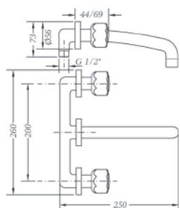
Ref.: 68131 11 45 66 Grupo de lavabo empotrado Built-in wash-basin
