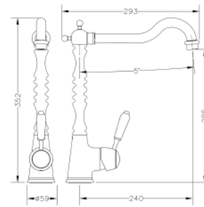
Ref.: 68201 39 43 66 Monomando de fregadera bronce Bronze sink mixer
