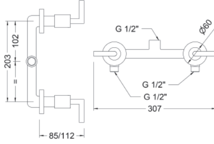
Ref.: 68115 12 45 66 Grupo ducha empotrado 8\"/>
