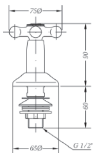
Ref.: 68520 09 45 66 Grifo bidé Bidet tap
