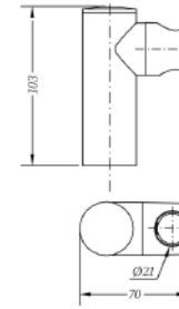
Ref.: 100153 45 Soporte ducha cilíndrico Cylindrical shower holder
