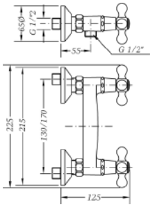
Ref.: 68530 09 45 66 Mezclador de ducha con kit Shower mixer with kit
