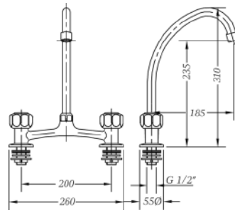
Ref.: 68199 11 45 66 Mezclador mesada 8" caño tubo 8" deck mixer with swan neck spout
