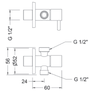
Ref.: 3107 04 Válvula de escuadra doble 1/2" - 1/2" ducha- inodoro Double angle valve 1/2" - 1/2"
