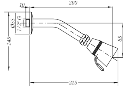
Ref.: 1698 45 Rociador ducha con brazo Wall shower arm and spray
