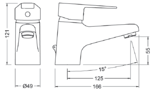
Ref.: 61130 28 45 66 Monomando de lavabo Plus Single lever Plus wash-basin mixer
