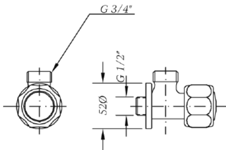
Ref.: 568083 45 Cuerpo grifo mural Wall body tap
