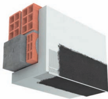
Traditerm® Perfil Goterón PVC con Malla
