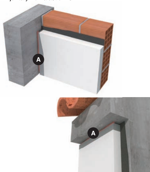
Detalles de aplicación fondo de junta + Pumalastic MS (A)
