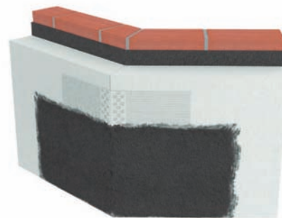
Traditerm® Perfil Ángulo Circular
