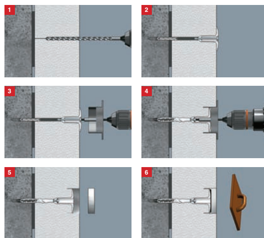
Método Interior Aislante
