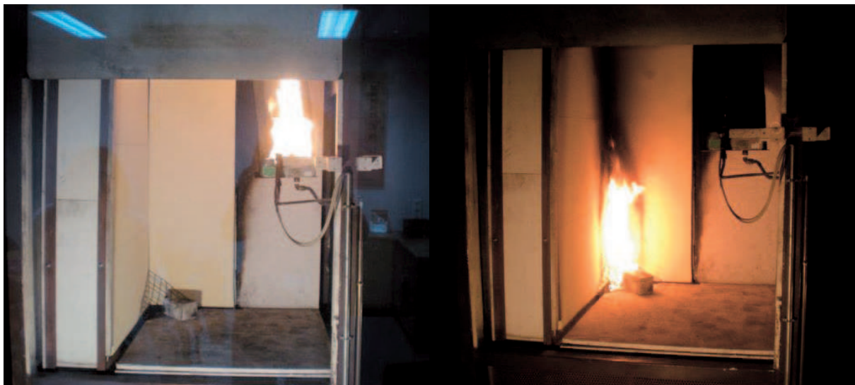
Ensayo de comportamiento frente al fuego
