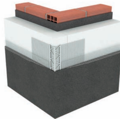
Traditerm® Perfil Ángulo PVC con Malla
