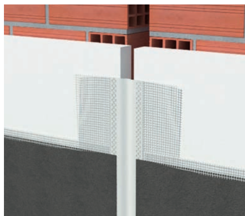
Traditerm® Perfil Junta Dilatación
