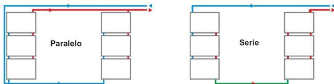
Figura 56: Formas de conexionado de dos baterías de captadores
