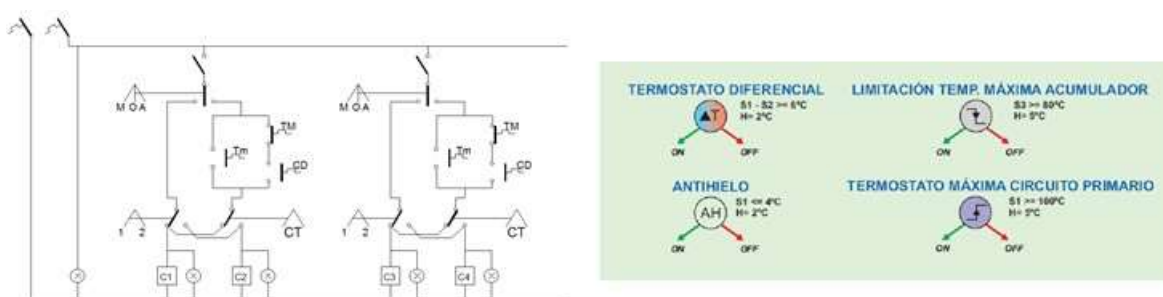
Figura 86: Izq.: Esquema eléctrico de alimentación a bombas en paralelo. Der.: Elementos de regulación de los valores de consigna del sistema de control y protección de una instalación solar
