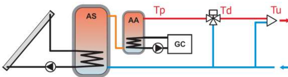
Figura 4: Temperaturas en una instalación de producción de ACS
