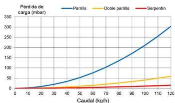
Figura 26: Pérdida de carga de tres tipos de absorbedor
