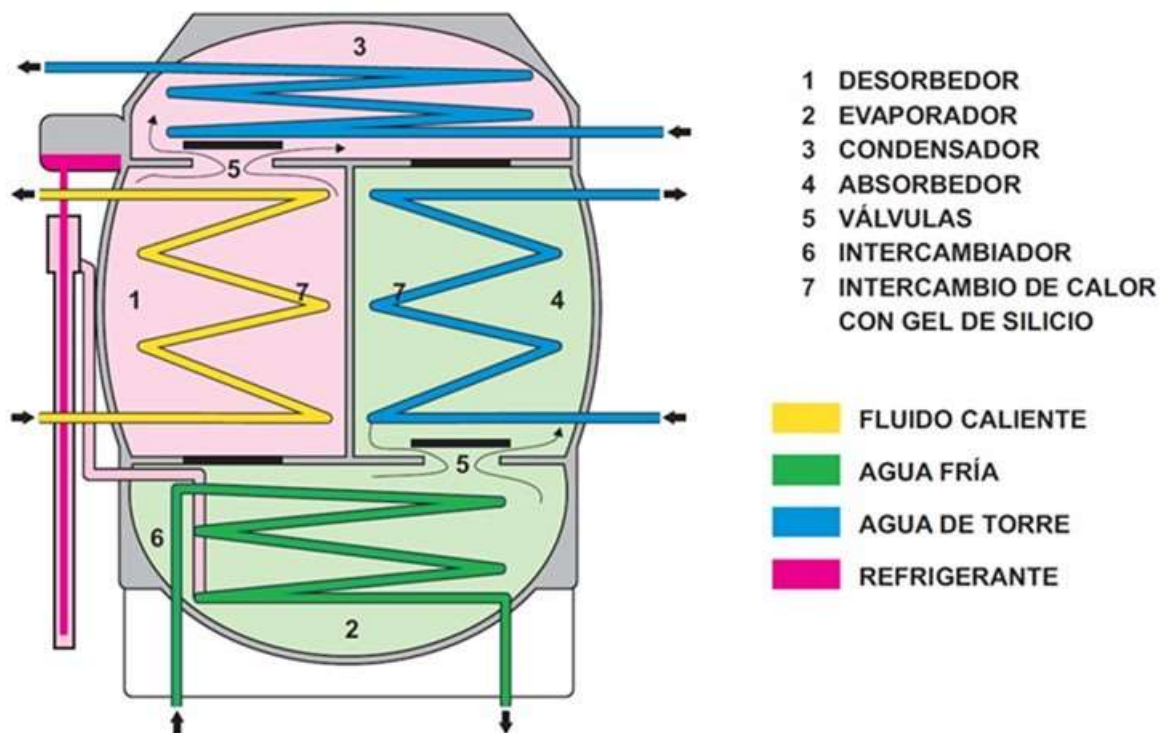
Figura 121: Esquema de un sistema de adsorción
