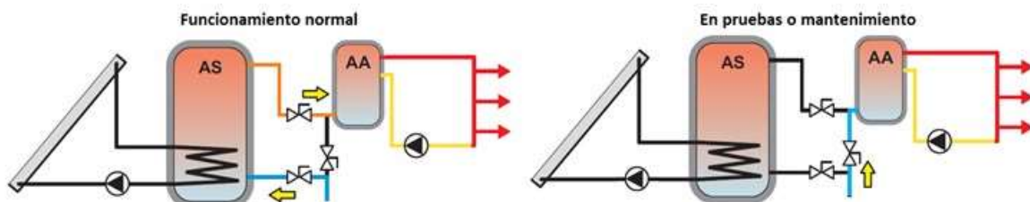
Figura 103: Actuación de las válvulas del bypass de alimentación en funcionamiento normal y en mantenimiento
