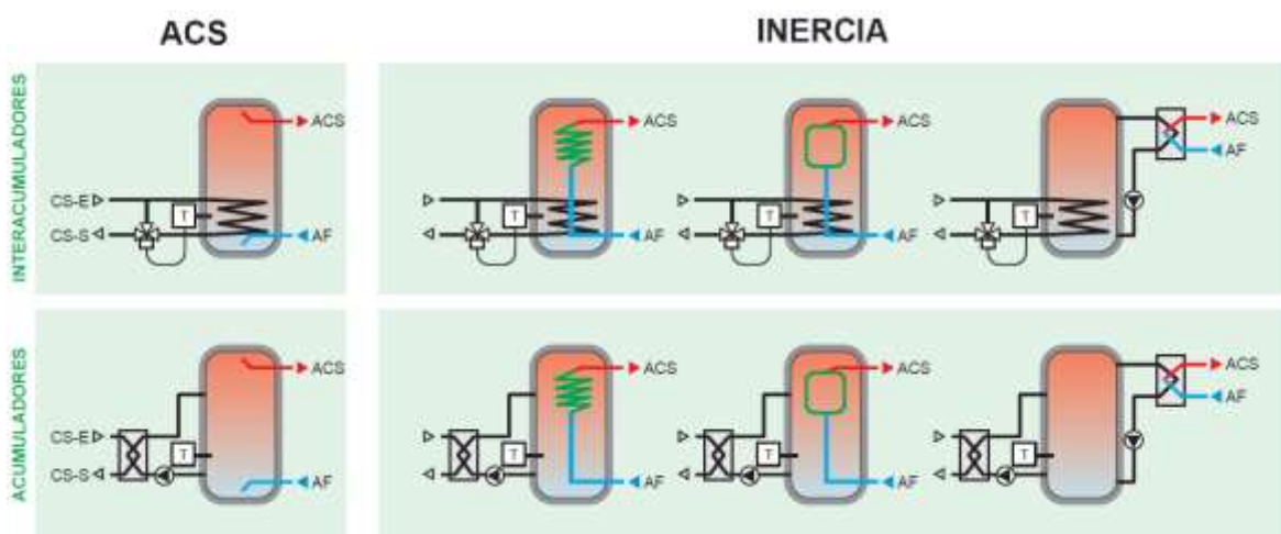
Figura 28: Diversos tipos de acumuladores e interacumuladores de ACS y de inercia
