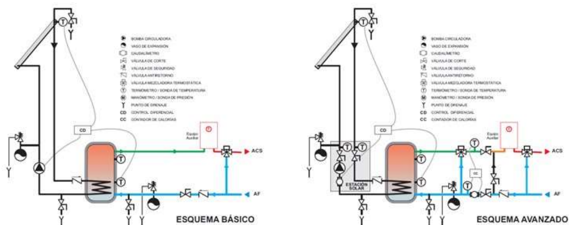
Figura 88: Esquemas y componentes de los esquemas básico (izquierda) y avanzado (derecha)
