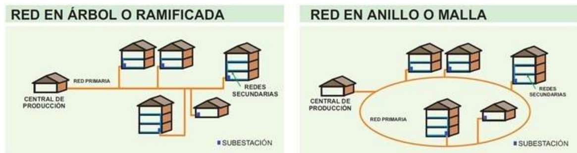
Figura 132: Dos formas de configurar el sistema de distribución de energía térmica
