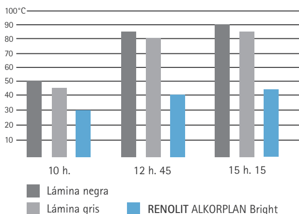
Temperatura con lámina impermeable de color negro Superficie de la cubierta 85 °C Interior del edificio 30 °C
