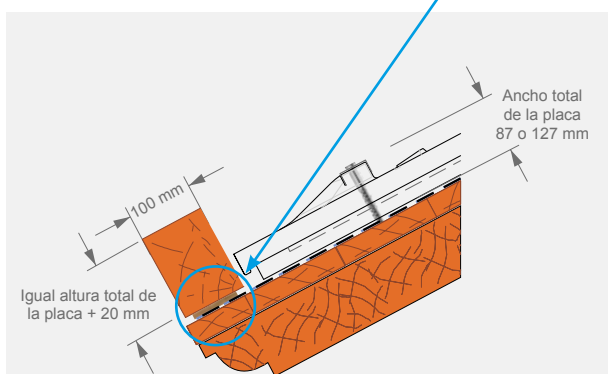
CON PEINE DE ALERO
