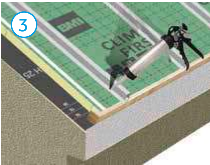
3. Sellado con adhesivo de poliuretano
