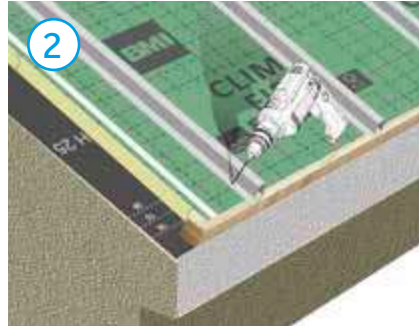
2. Perforación de rastrel, panel y forjado
