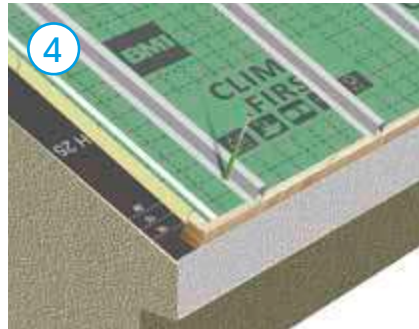
4. Introducción de taco de impacto
