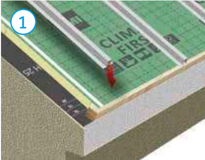
1. Replanteo rastrel primario (distancia 50 cm.)
