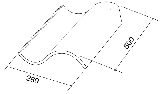
TEJA VEREA SPANISH S DE ALERO
