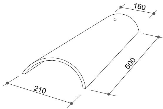
TEJA CURVA FINAL IZQUIERDO
