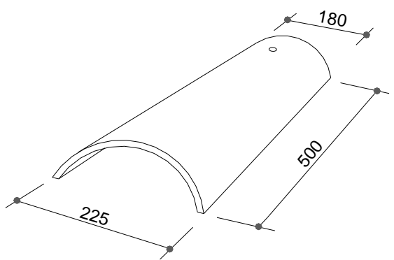
TEJA DE CUMBRERA
