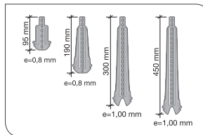
CUELGUE P 11-21-31-41T-45
