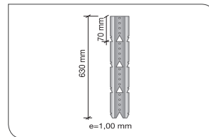
CUELGUE PF 61-T-45
