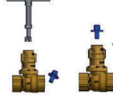
6 Extraer la llave y introducir el tapón de protección. La válvula permanecerá bloqueada (en 10% apertura). / Remove the key and insert the plastic protection cap. The valve will remain locked (at 10% opening).
