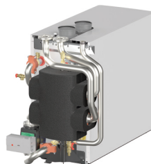
Kit botella de equilibrio Profundidad del kit 407 mm. Ida/retorno DN50. Conexión gas 1 1/2".
