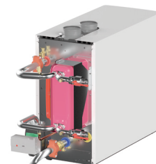
Kit intercambiador de placas Profundidad del kit 639 mm. Ida/retorno 2". Conexión gas 1 1/2".
