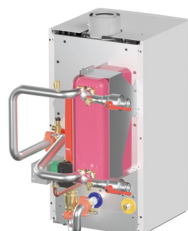
Kit intercambiador de placas Profundidad del kit 634 mm. Ida/retorno 1 1/2". Conexión gas 1".
