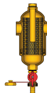
Esquema montaje accesorio: Desfangador + Sep. Magnético
