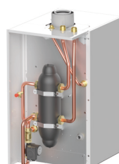
Kit botella de equilibrio Profundidad del kit 250 mm. Ida/retorno 1 1/2". Conexión gas 1".
