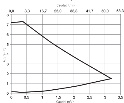
Curva del circulador incluido en modelos GT, GTF, GTA y GTF
