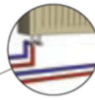
Sistema bitubo por colectores (dos tuberías desde el colector)
