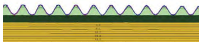
Distribución de isotermas a través de la solución con cámara de aire
