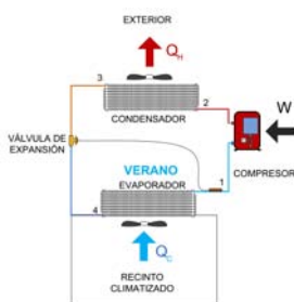
Esquema básico de sistema de climatización convencional en modo verano.
