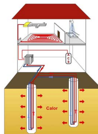
Esquema de captación cerrada vertical.
