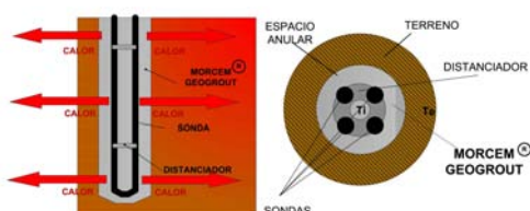
Esquema con Morcem®Geogrout
