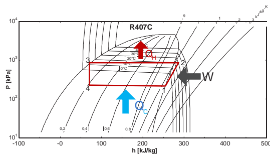
Ciclo de refrigerante. Trabajo de compresión 3-4 y condensación 4-1.
