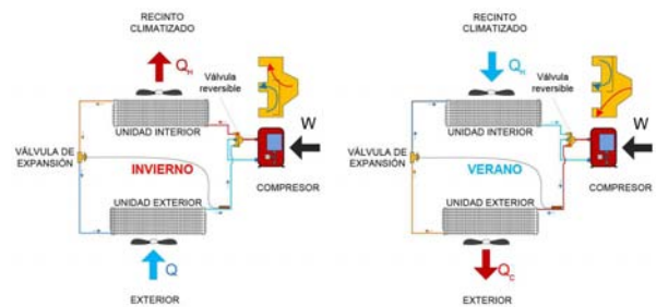
Inversión del ciclo mediante válvula inversora o cuatro vías. Modo de funcionamiento en régimen invierno y en régimen verano.
