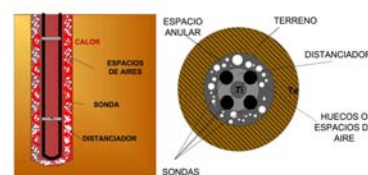
Esquema con gravas
