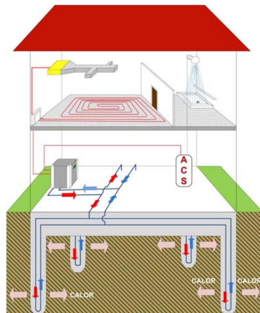
Esquema de captación mediante pilotes geotérmicos.
