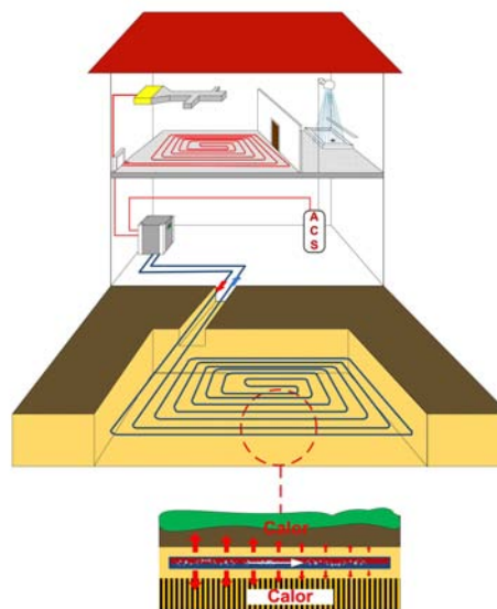
Esquema de captación cerrada horizontal.
