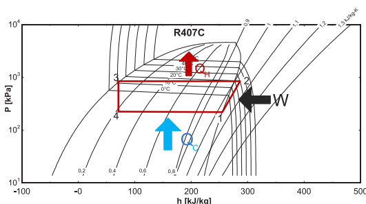
Ciclo de refrigerante. Trabajo de compresión 1-2 y condensación 2-3.
