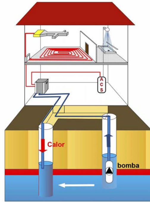
Esquema de captación en acuífero somero.
