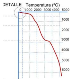
Gradiente Geotérmico típico en el subsuelo terrestre.
