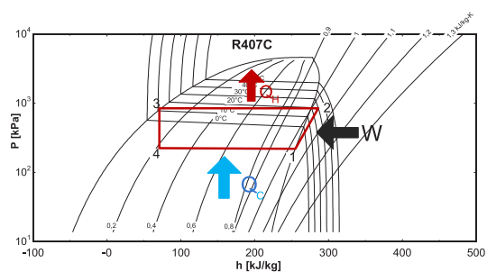
Ciclo de refrigeración en modo verano. Ciclo de refrigerante.
