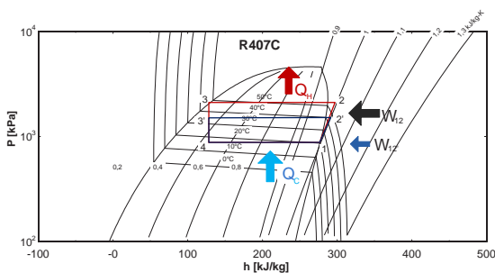
Ciclo de refrigerante. Disminución de trabajo de compresión mediante disminución en temperatura de condensación.
