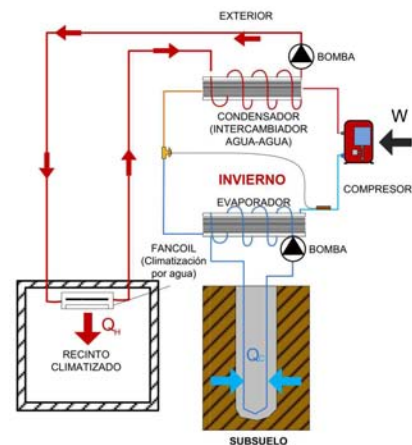
Esquema básico de una unidad geotérmica.
