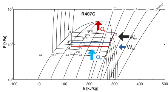
Ciclo de refrigerante. Disminución de trabajo de compresión mediante disminución en temperatura de calefacción.
