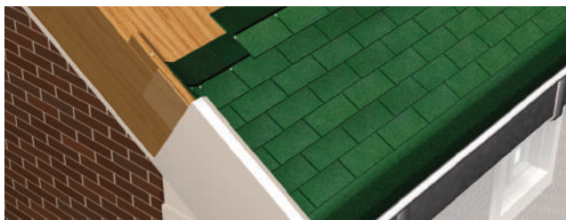
Remates con perfiles metálicos o piezas especiales (laterales)
