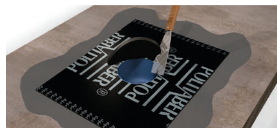
Perfilar el agujero a la cazoleta
