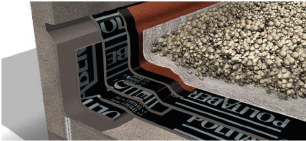
Cubierta convencional. No transitable, acabada con grava. Bicapa.
