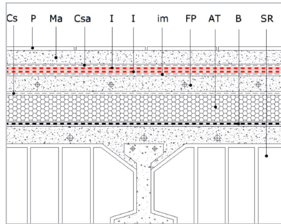
Cubierta plana convencional el aislamiento térmico XPS se sitúa debajo de la membrana impermeabilizante.
