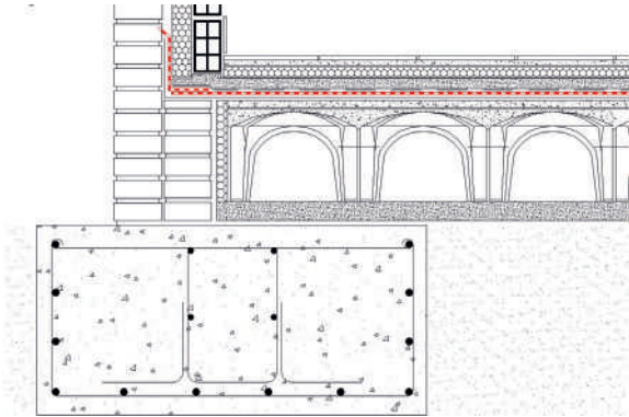
FORJADO CAVITI
