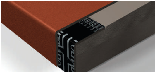
Arranque de la impermeabilización.
