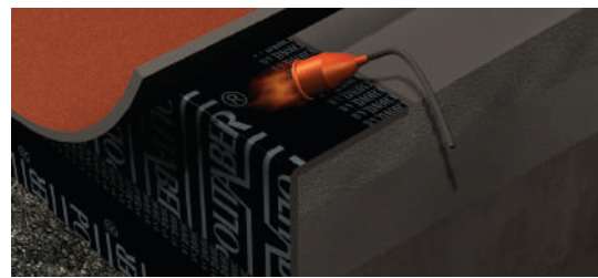
Aplicación pieza inicio.
