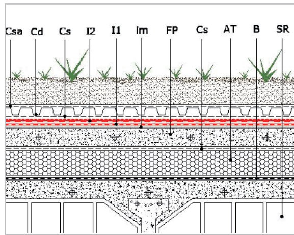
Cubierta plana convencional
